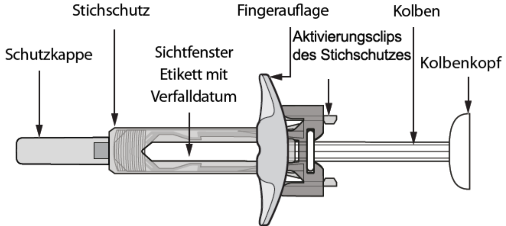
Abbildung A: Hyrimoz-Fertigspritze mit Stichschutz und Fingerauflage
