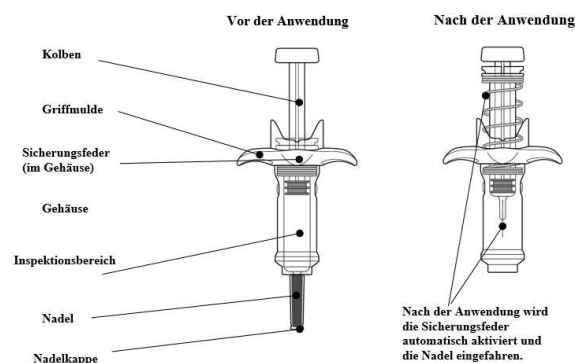
Bestandteile: Übersicht
